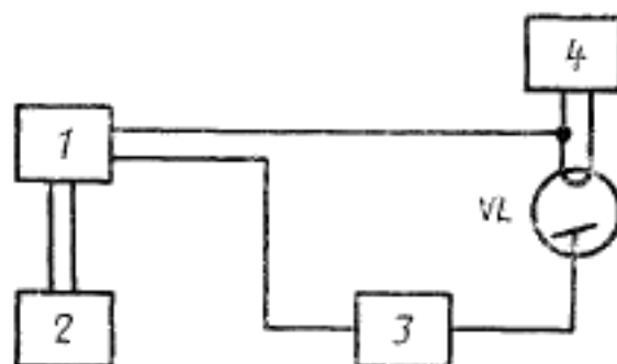
1 — управляемый источник напряжения swing-1000 В; 2 — устройство задания длительности прохождения тока рентгеновской трубки; 3 — измеритель количества электричества; 4 — источник питания накала. VL — рентгеновская трубка
